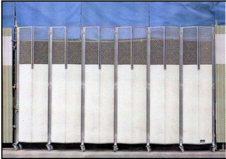
パネルキャスターゲート H=3m (PCGN)
