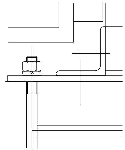
詳細 C 1/5
