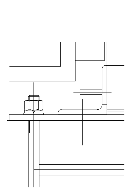
詳細 C 1/5
