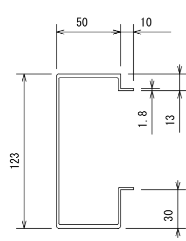
材質 A6N01S-T5 枠断面形状
