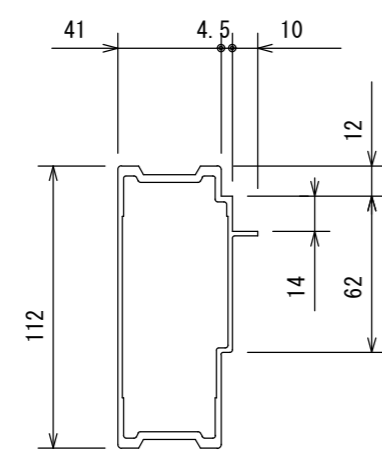
材質 A6N01S-T5 枠断面形状
