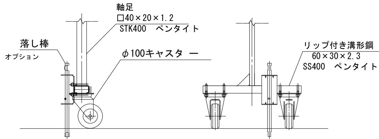
足廻り詳細
